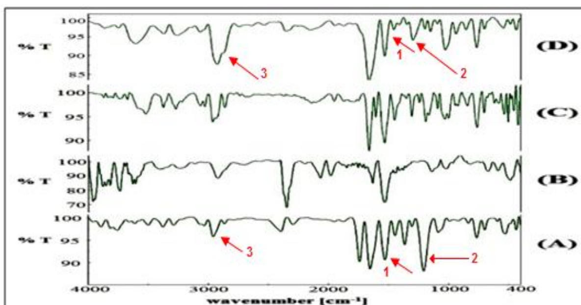
Fig. 1. IR spectra of (A) Pure LPO (B) \beta CD (C) PM (D) SD-MWI
