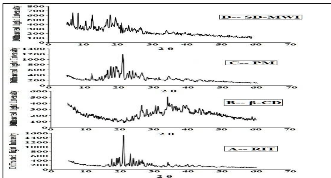
Fig. 6. XRD profile of (A) LPO (B) β-CD (C) PM (D) SD-MWI
